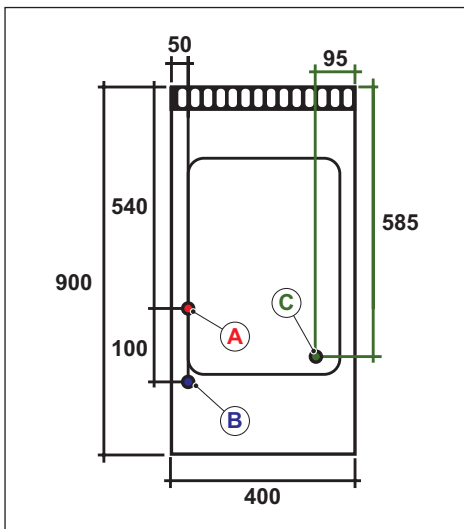
Fig. 13 Una vasca
