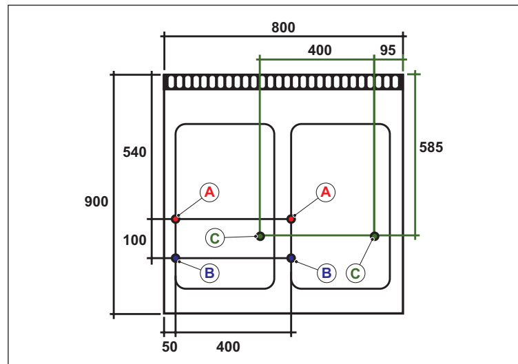
Fig. 14 Due vasche
