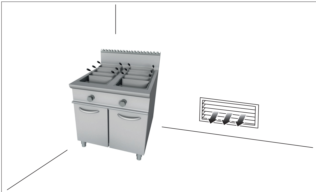
Fig. 18 Ventilazione del locale di installazione
