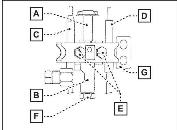
Fig. 24 Parti principali dell'ugello pilota
