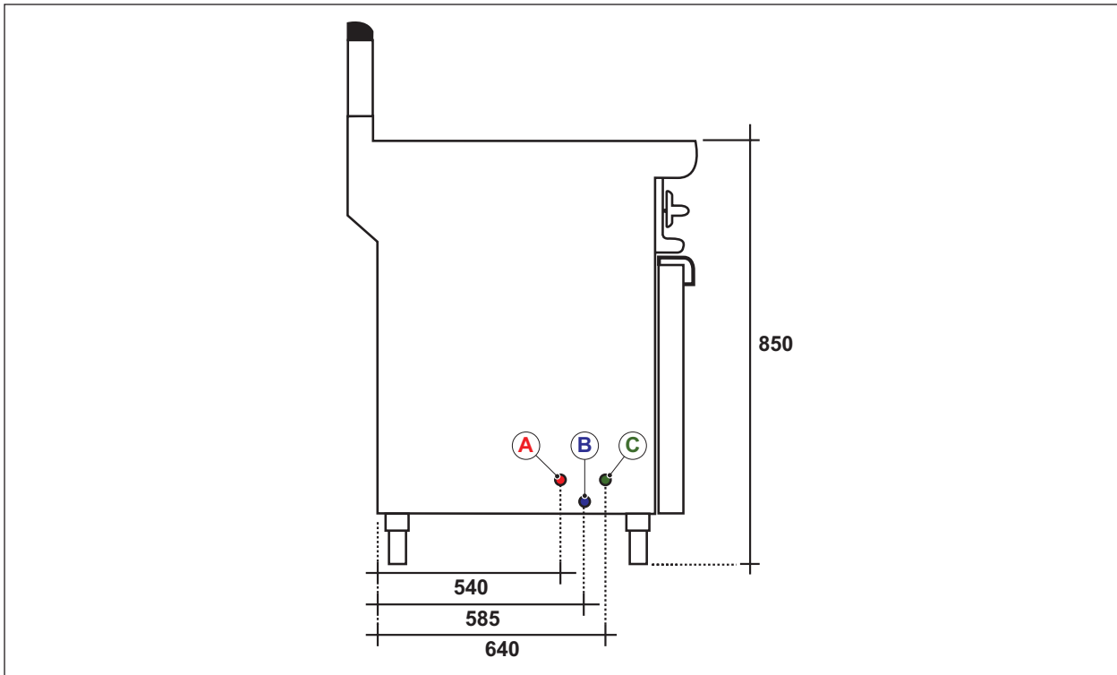
Fig. 12 Dimensioni cuocipasta
