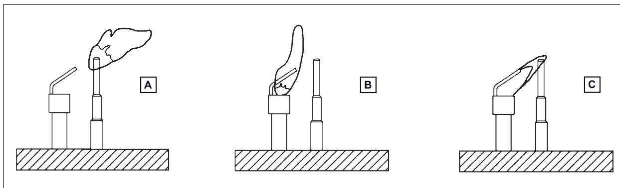
Fig. 21 Regolazione della fiamma pilota
