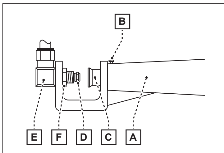
Fig. 22 Parti principali del bruciatore
