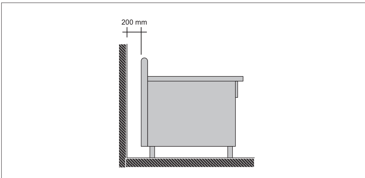
Fig. 17 Distanza minima da pareti infiammabili
