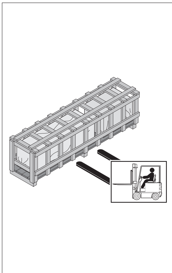
Fig. 11 Imballaggio
