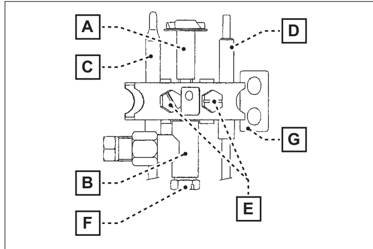
Fig. 23 Parti principali dell'ugello pilota
